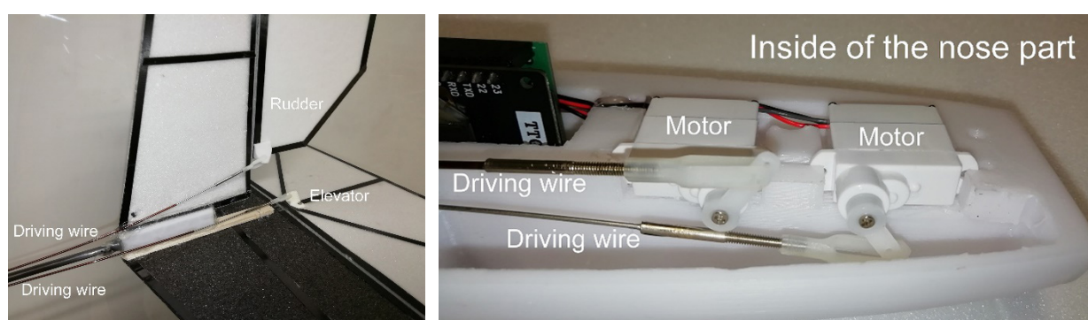
図2 フィードバック制御系の実現（モータドライバ、モータ、リンク、駆動ワイヤー）
