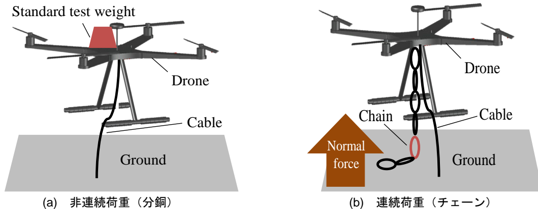
図 11 ペイロード検証実験の方法
