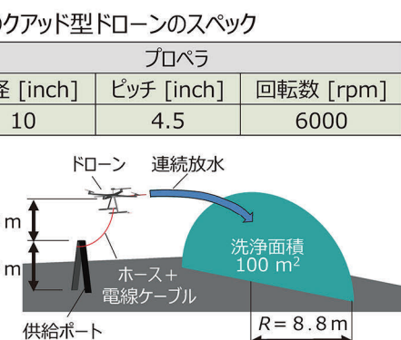
図3. 連続放水飛行の概略と放水面積
