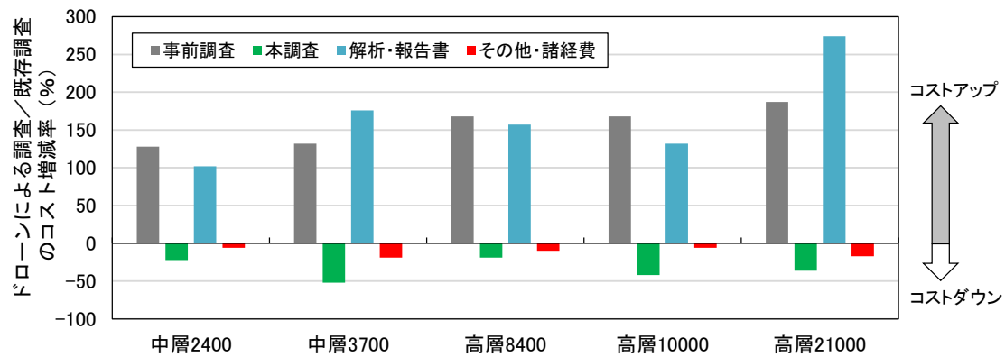
図 14 12 条点検において既存調査を基準とした場合のドローンによる外壁調査の分類別コスト増減率
